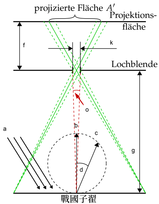
Figure 1: Ein Lambertreflektor reflektiert einfallendes Licht
